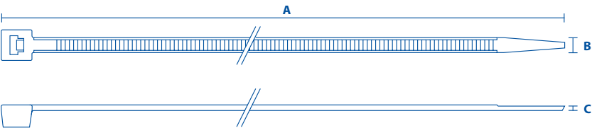
CARACTERÍSTICAS DIMENSIONALES
