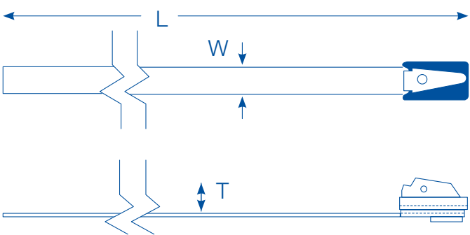
CARACTERÍSTICAS DIMENSIONALES
